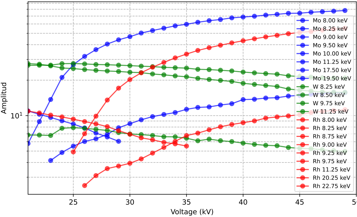
Amplitud vs Voltage
